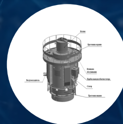
Электродвигатель ГЦНА-1753
